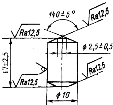
Конструкция и размеры шипа D_a = 10 мм
