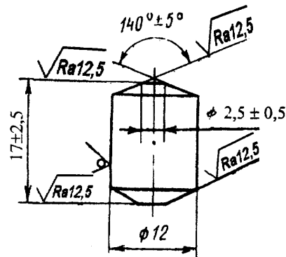
Конструкция и размеры шипа D_a = 12 мм
