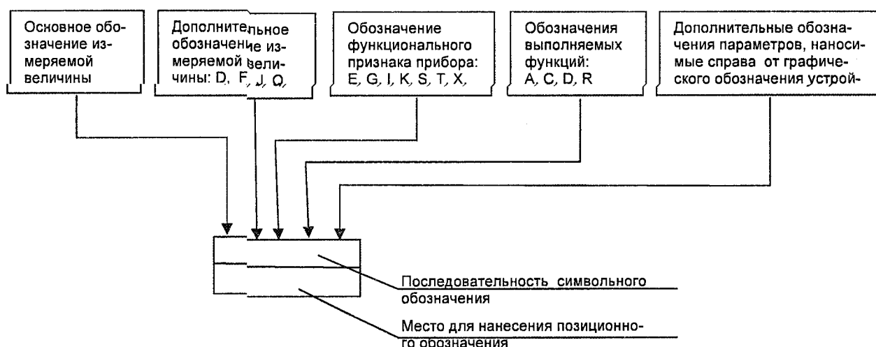
Рисунок 1 — Принцип построения условного обозначения прибора
