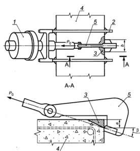
Рисунок Б.1. Схема испытания методом скалывания ребра"
