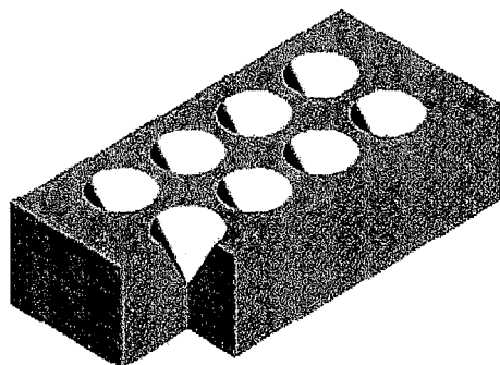
Рисунок А.3 — Изделие с несквозными пустотами
