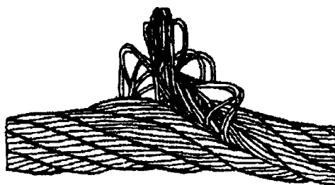
Рисунок 11. Выдавливание сердечника.
