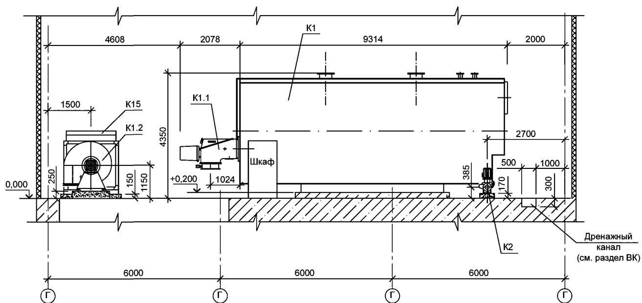
Рисунок А.2 - Пример выполнения разреза расположения оборудования
