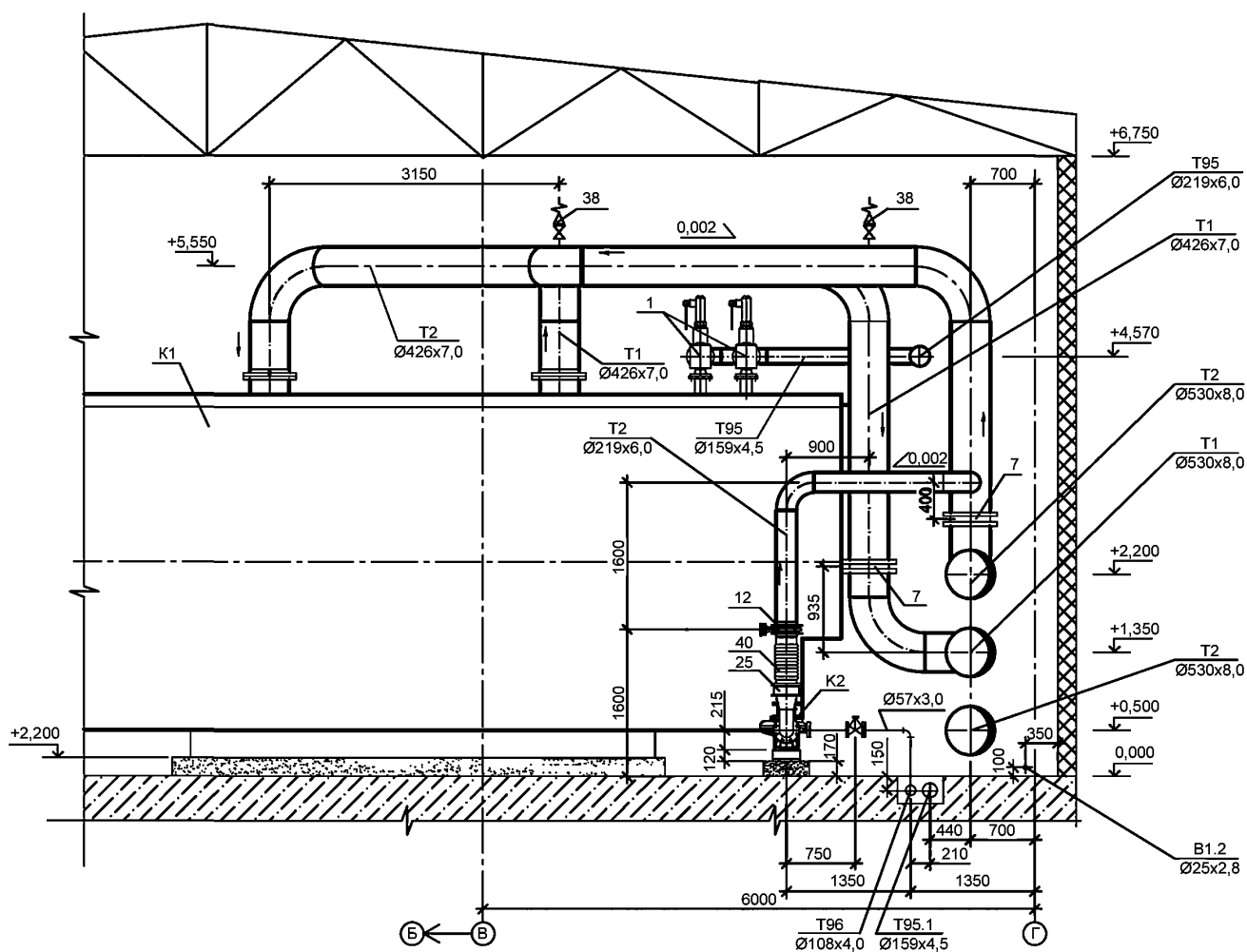
Рисунок В.2 - Пример выполнения поперечного разреза расположения трубопроводов
