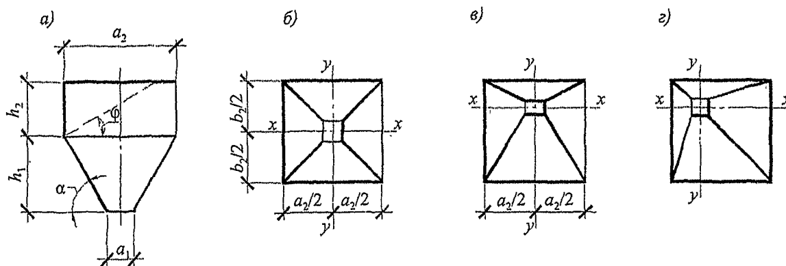
а – схема бункера; б – симметричный пирамидальный бункер; в – частично симметричный пирамидальный бункер; з – несимметричный пирамидальный бункер
