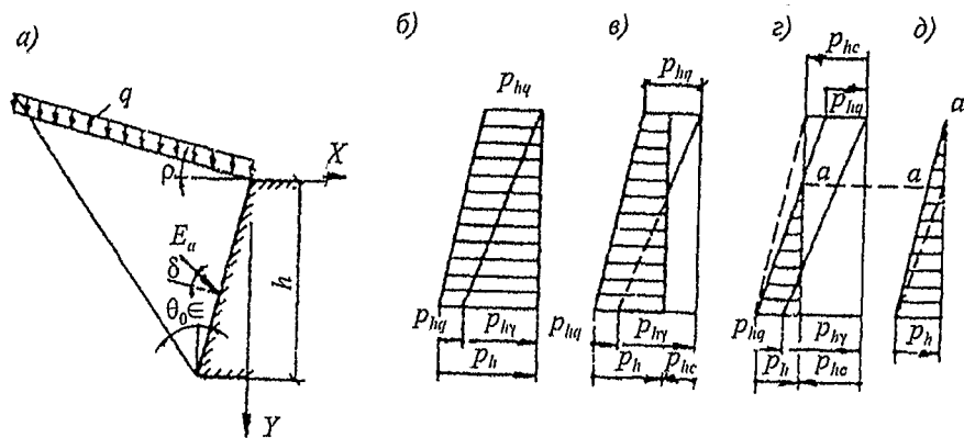
a – на стену; b – при отсутствии сцепления p_{hc}=0 ; c – при p_{hc} < p_{hq} ; d – при p_{hc} \geq p_{hq} ; d – заменяющая (расчетная) эпюра
