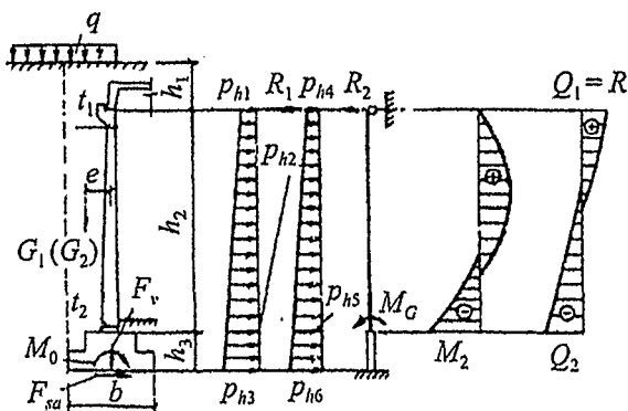
Рисунок 3 – Расчетная схема стены подвала
