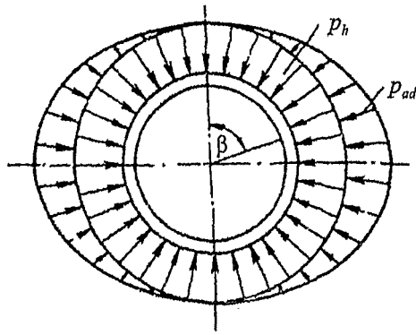
Рисунок 5 – Схема распределения основного p_h и дополнительного p_{ad} горизонтального давления грунта на круглый колодец
