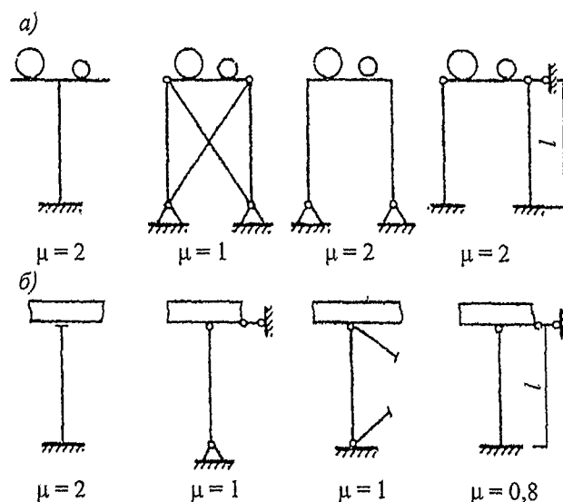
Рисунок 11 – Значения коэффициентов для определения расчетных длин l_0 = \mu l колонн опор
