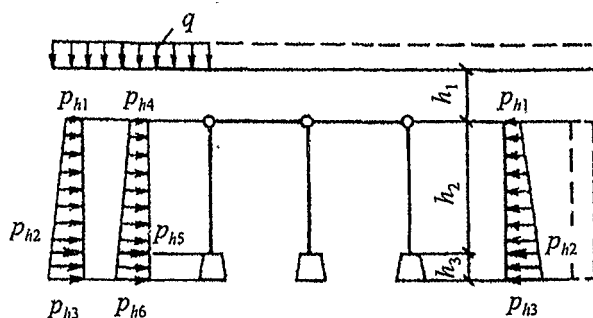
Рисунок 2 – Расчетная схема поперечной рамы подвала
