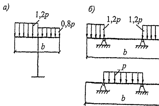
Рисунок 8 – Распределение интенсивности вертикальной нагрузки при расчете траверс отдельно стоящих опор и эстакад
