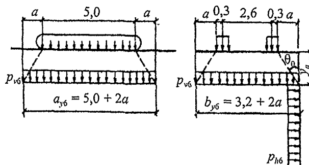
Рисунок B.6 – Схема давления от гусеничной нагрузки НГ-60 при движении ее вдоль сооружения
