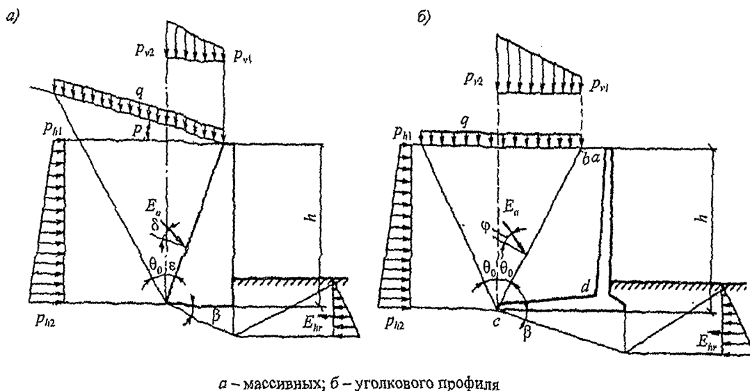
Рисунок 1 – Расчетные схемы подпорных стен
