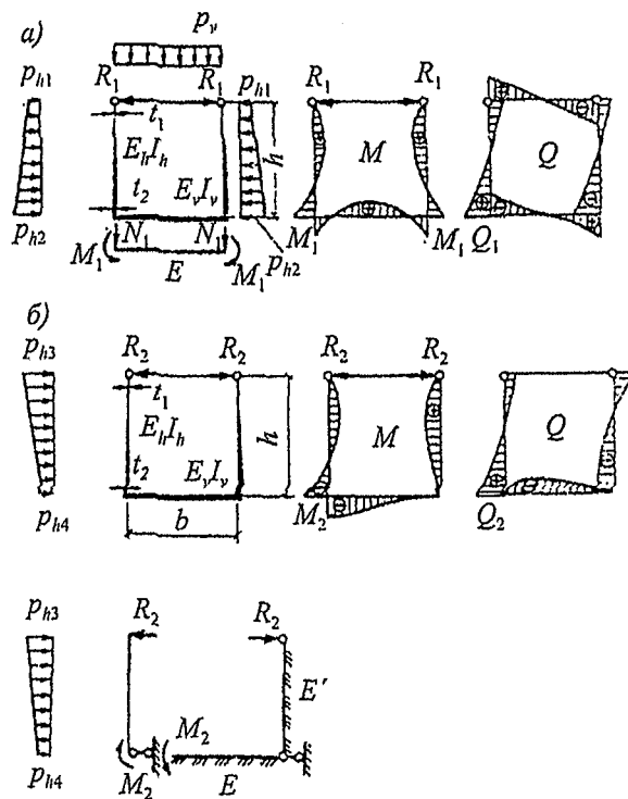
а – симметричное нагружение; б – одностороннее нагружение
