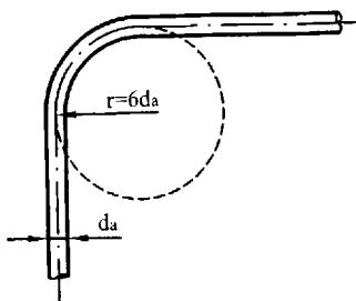
Рисунок 13 — Холодная гибка медной трубы
