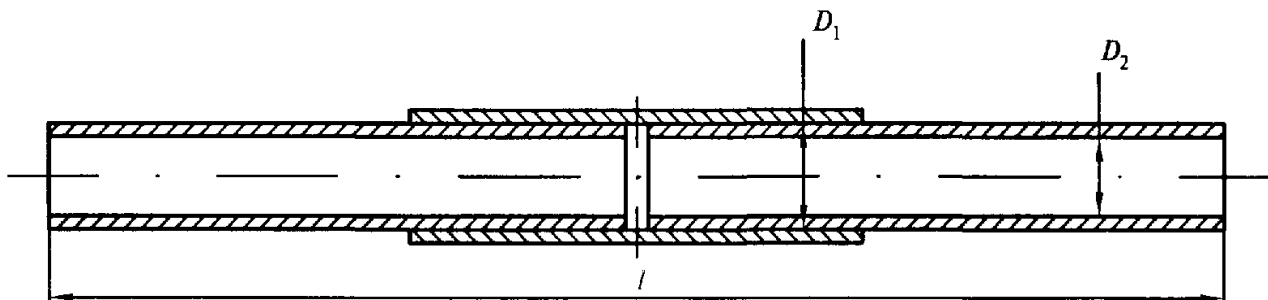
Рисунок 8 — Допускное соединение
