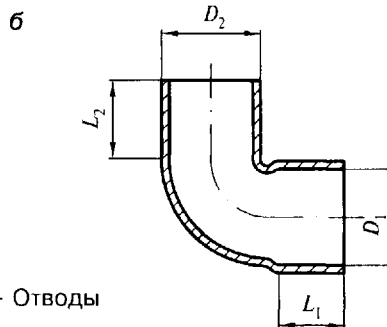
б — с раструбным и гладким концами
