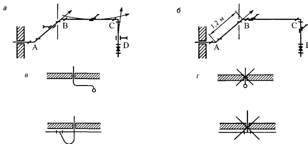
Рисунок 7 — Прокладка газопроводов с соблюдением правил естественной компенсации
