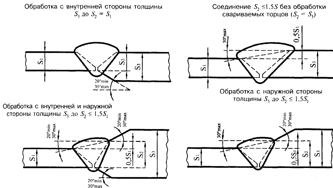
Рисунок 10 — Обработка свариваемых торцов труб
