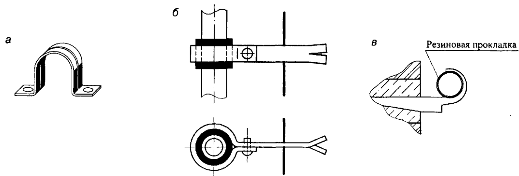
Рисунок 5 — Опоры для крепления медных газопроводов
