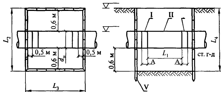
Рисунок Л.1 — Вставка стальной катушки
