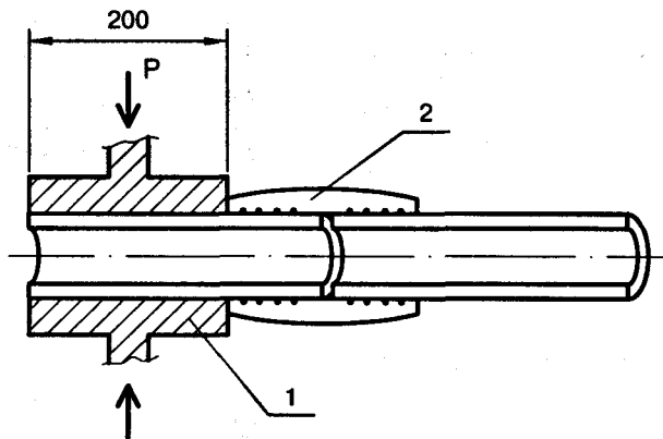
Рисунок Т.2 — Схема испытания образцов-сегментов на сплющивание
