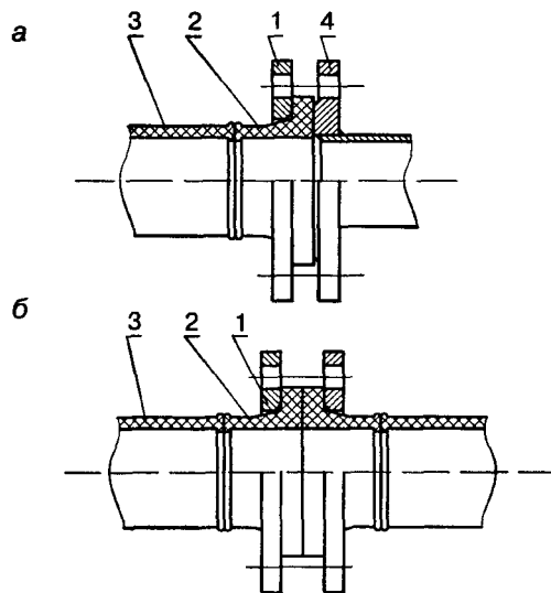
а — полиэтиленовых труб со стальными трубами, арматурой; б — полиэтиленовых труб между собой; 1 — фланец стальной свободный; 2 — втулка под фланец из полиэтилена; 3 — труба из полиэтилена; 4 — фланец стальной трубы, арматуры
