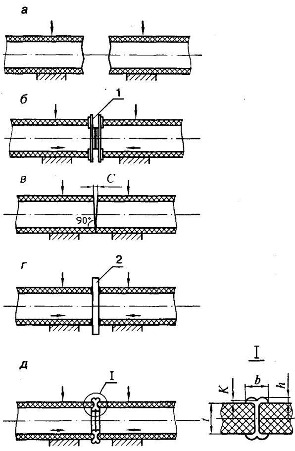
а — центровка и закрепление в зажимах сварочной машины концов свариваемых труб; б — механическая обработка торцов труб с помощью торцовки 1 ; в — проверка соосности и точности совпадения торцов по величине зазора С ; г — оплавление и нагрев свариваемых поверхностей нагретым инструментом 2 ; д — осадка стыка до образования сварного соединения (в сечении I даны буквенные обозначения основных геометрических размеров соединения встык, регламентированные, 8.11, 8.12, таблицей 23 настоящего СП)
