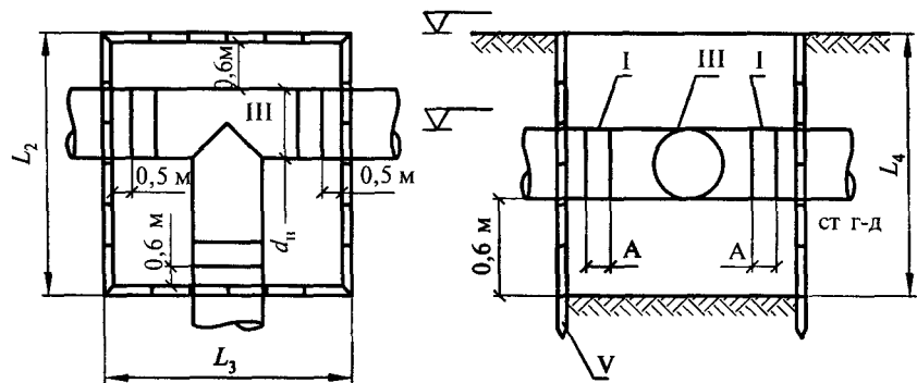
Рисунок Л.2 — Вставка тройника
